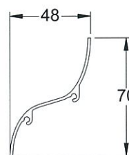
Fin type 6 Material: Aluminium
