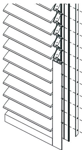
Fin type 4 Material: Aluminium
